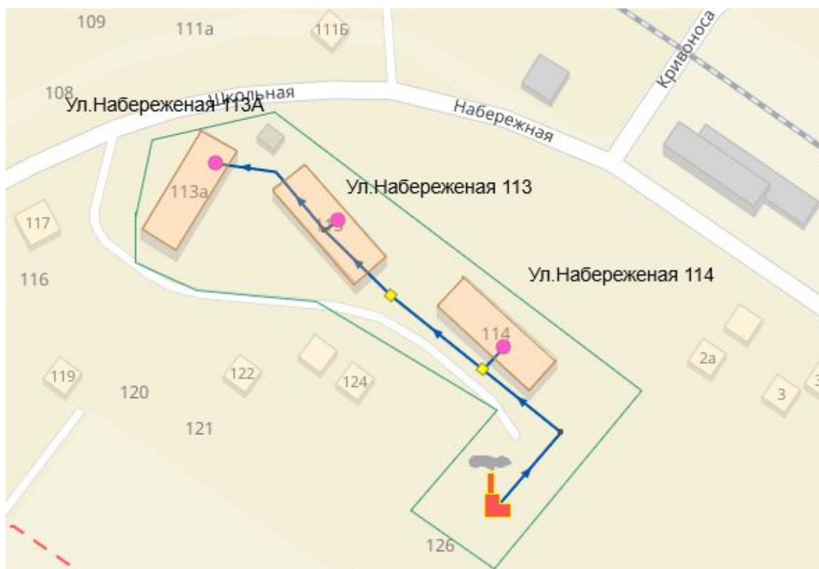
Рисунок 6.2.1 - Существующая трассировка тепловых сетей
